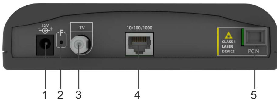
Рисунок 4 — Внешний вид задней панели NTU-1C
