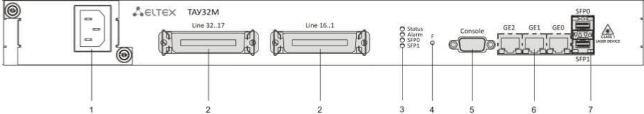
Рисунок 7 – Внешний вид передней панели TAU-32M.IP
