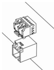
Рисунок 26 — Установленные SFP-трансиверы
