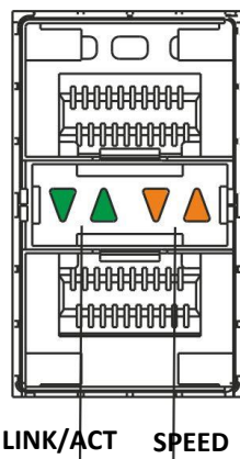
Рисунок 20 — Внешний вид разъема с SFP-трансиверами
