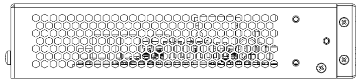
Рисунок 50 – Левая боковая панель MES2300-24, MES2300B-24, MES2300-24P
