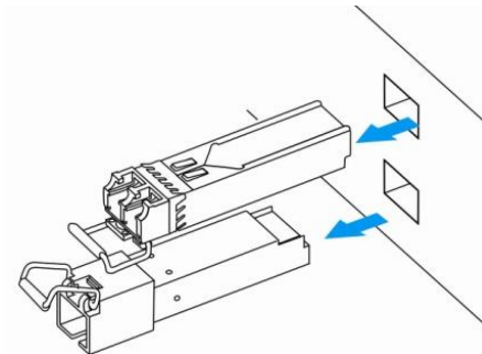
Рисунок 86 – Извлечение SFP-трансиверов
