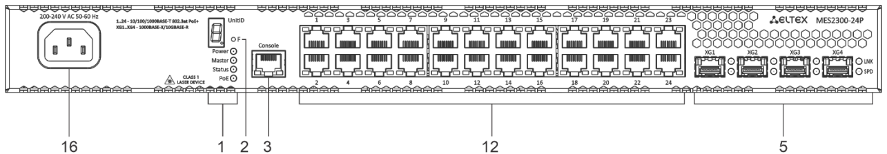
Рисунок 8 – Передняя панель MES2300-24P
