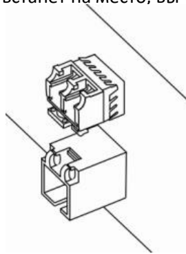
Рисунок 84 – Установленные SFP-трансиверы
