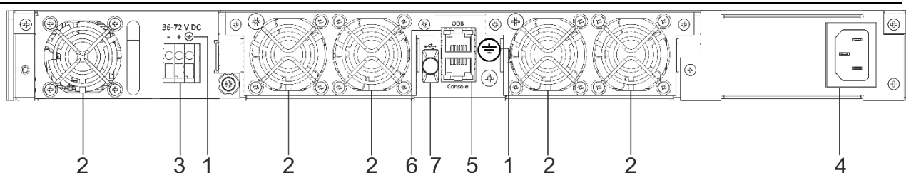
Рисунок 47 – Задняя панель MES5400-48
