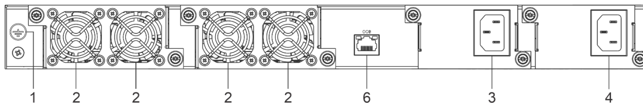
Рисунок 41 – Задняя панель MES3300-48, MES3300-48F
