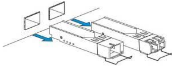
Рисунок 14 – Извлечение SFP-трансиверов
