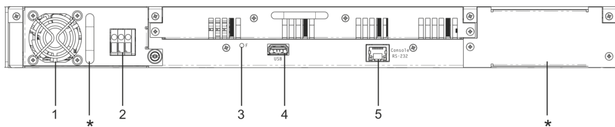
Рисунок 3 - MES5148 задняя панель 2
