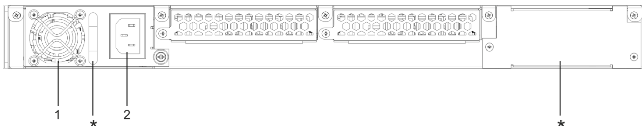
Рисунок 4 - MES5248 задняя панель 1
