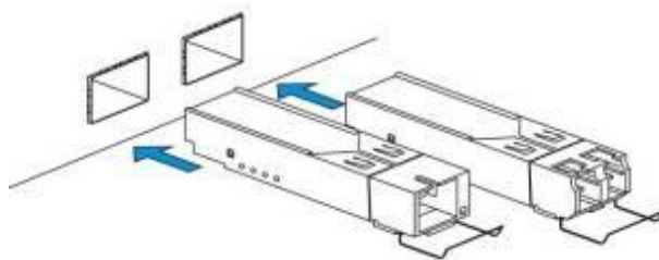
Рисунок 11 – Установка SFP-трансиверов
