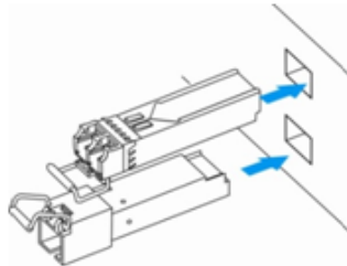
Рисунок 23– Установка SFP-трансиверов
