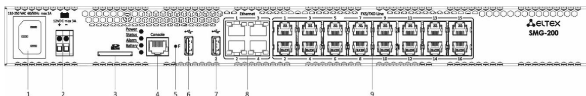
Рисунок 6 — Внешний вид передней панели SMG-200
