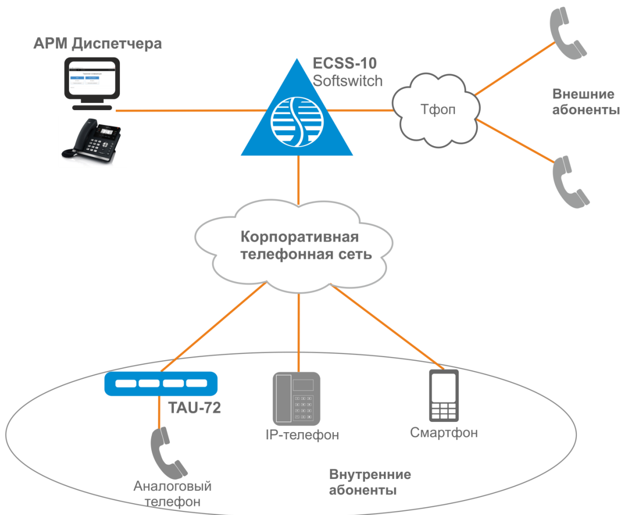
Рисунок – Система корпоративной и селекторной связи ECSS-10
