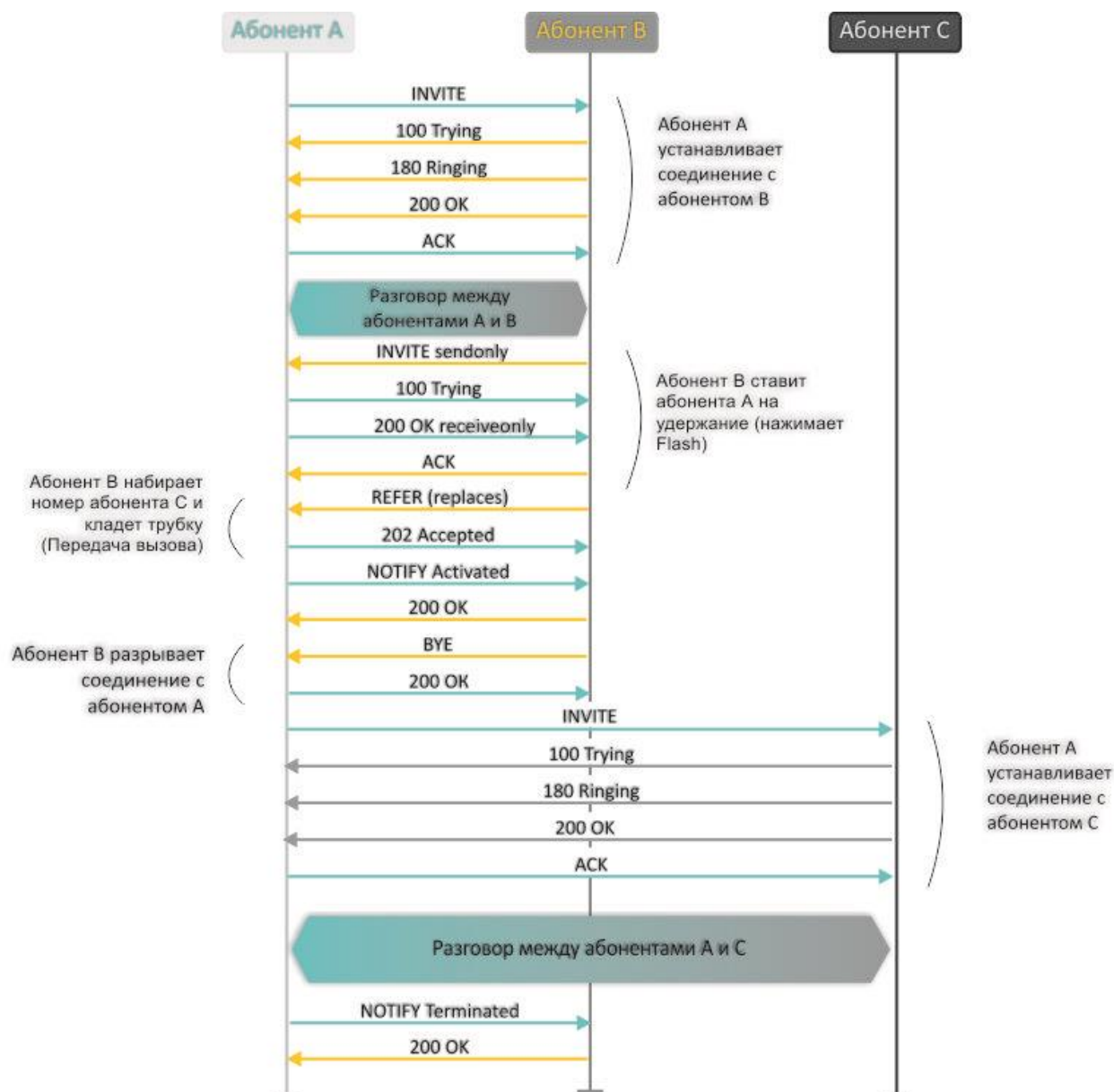
Рисунок 7 – Алгоритм работы услуги «Unattended calltransfer»
