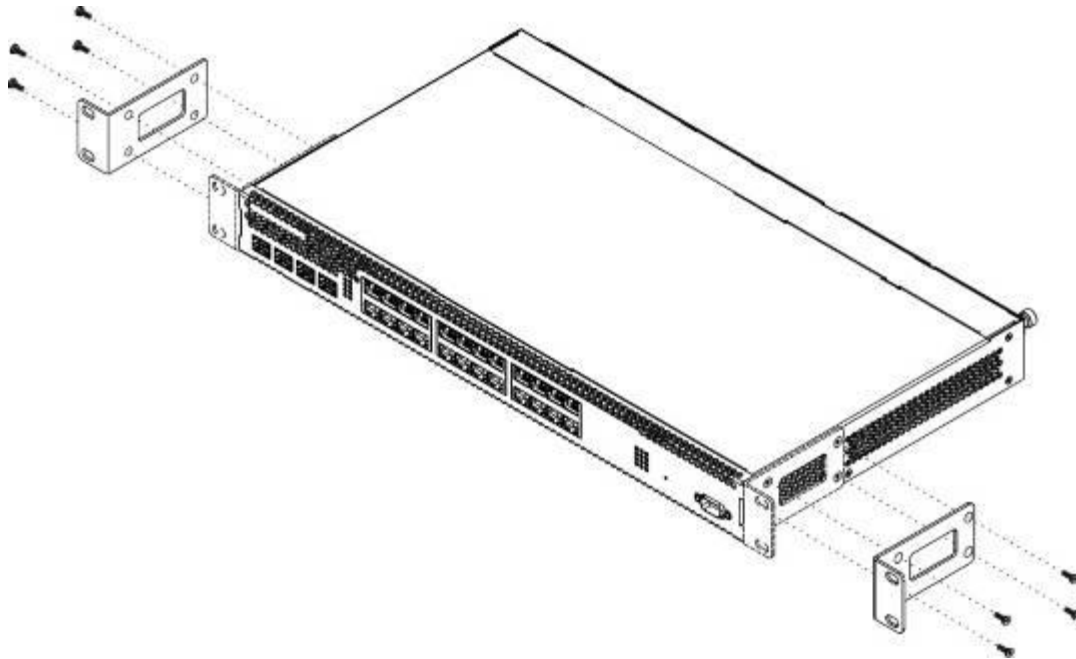
Рисунок 15 – Крепление кронштейнов
