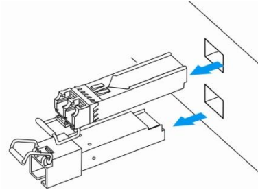
Рисунок 22 – Извлечение SFP-трансиверов
