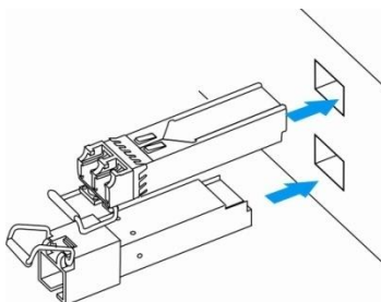
Рисунок 19 – Установка SFP-трансиверов
