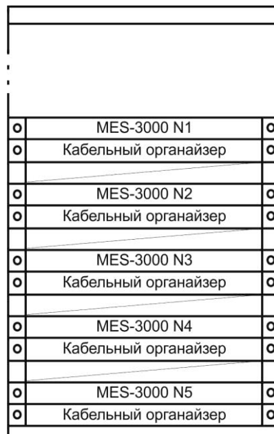
Рисунок 17 – Размещение коммутаторов MES3000 в стойке
