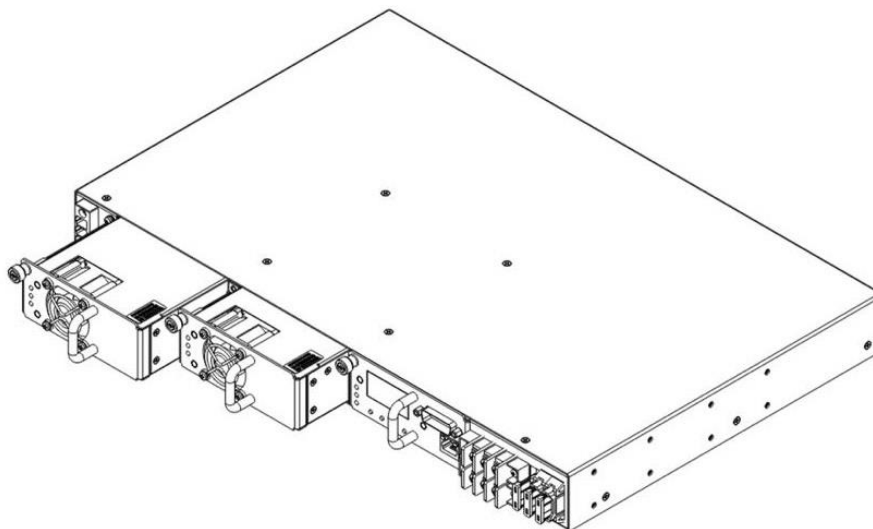
Рисунок 5 – Установка модулей питания
