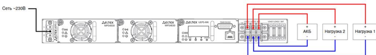
Рисунок 8 – Схема включения УЭП5-2
